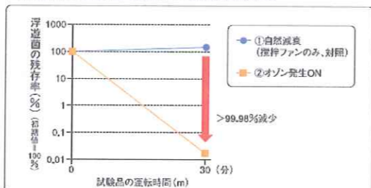
クワカワカビ (胞子) に対する試験結果 (初期値=100%)
