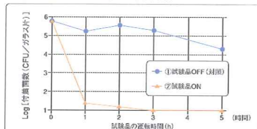
ガラス片付着菌に対する試験結果
